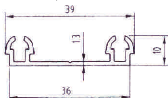
PVC GUIDE
