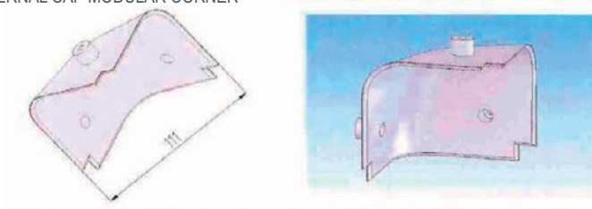
Roh k rohové liště – vnitřní 3 WAY INTERNAL CAP MODULAR CORNER
