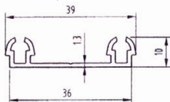
PVC GUIDE
