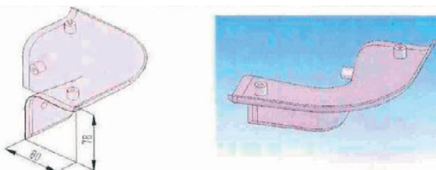
Roh k rohové liště – vnější 3 WAY EXTERNAL CAP MODULAR CORNER
