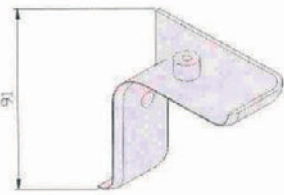
Krytka narážecí lišty END CAP MODULAR BUMPER
