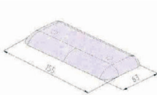
Krytka narážecí lišty END CAP MODULAR BUMPER
