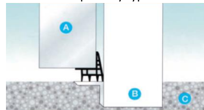
Práh v úrovni podlahy typ S2:
